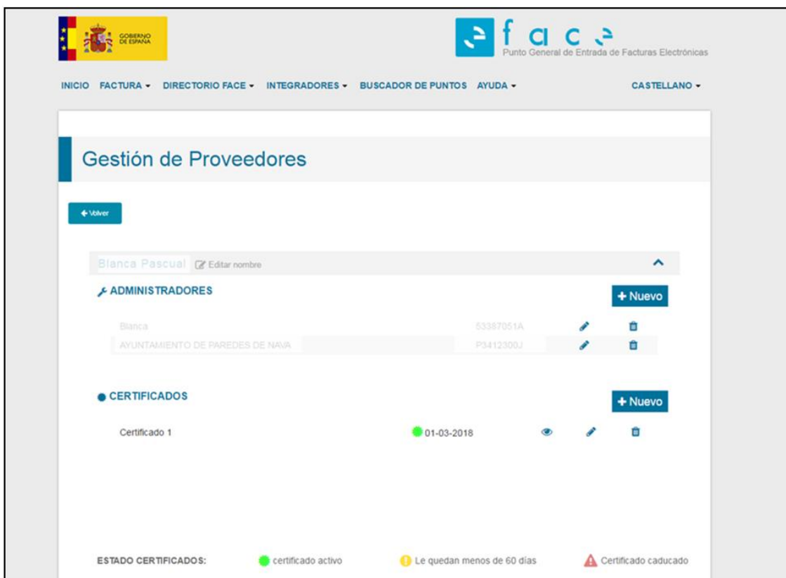
Ilustración 27. Gestión proveedores
