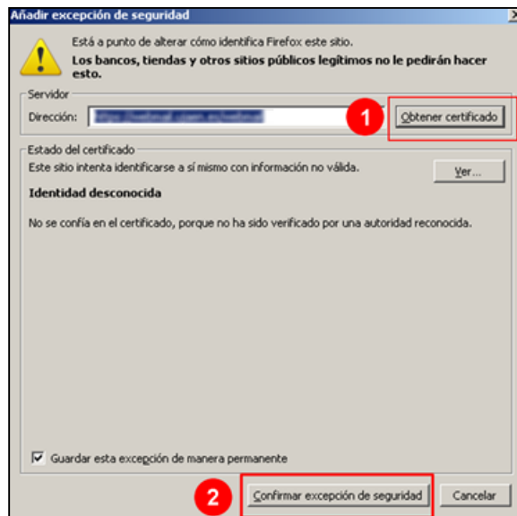
Ilustración 38. Añadir excepción
