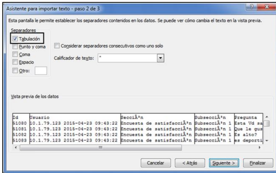
Ilustración 34. Seleccionar tabulador
