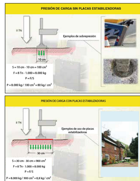
Figura 25. Presión de carga ejercida sobre la superficie de apoyo con y sin placas estabilizadoras.
